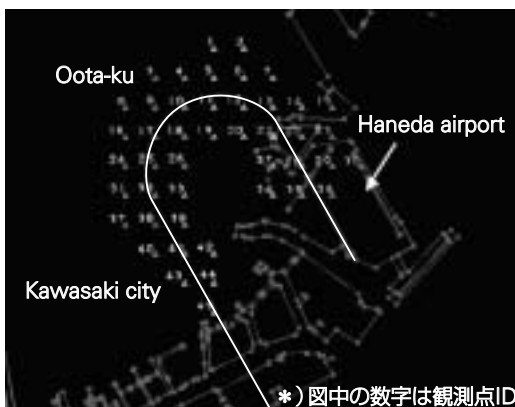
■図—6 B767による65+dB(A)騒音暴露地域
