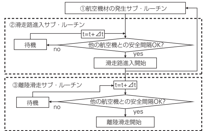
■図—4 離陸機のメイン・ルーチン
