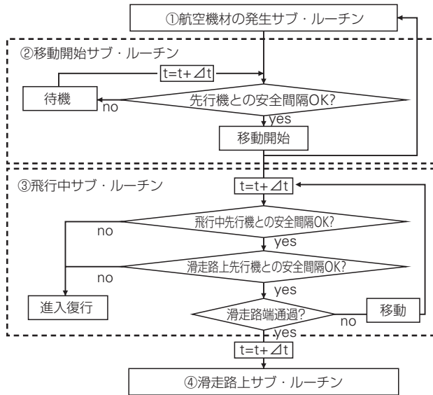
■図—3 着陸機のメイン・ルーチン
