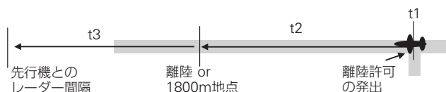
■図一2 離陸機を処理するための時間の区分
